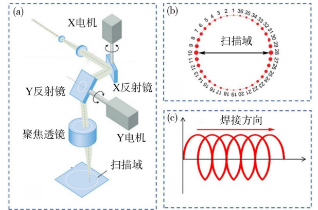
图2 FDPM-LW模式示意:(a)设备;(b)功率设置;(c)扫描轨迹
