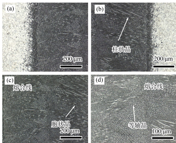
图 9 GHS-LW 焊缝表面金相组织: (a) 焊缝左侧; (b) 焊缝右侧; (c) 焊缝中心; (d) 焊缝中心等轴晶
