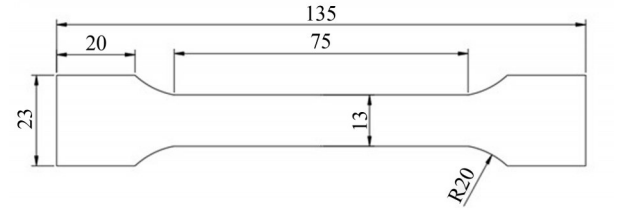
图4 拉伸试样尺寸示意(单位:mm) Fig. 4 Size diagram of tensile specimen (unit: mm)
