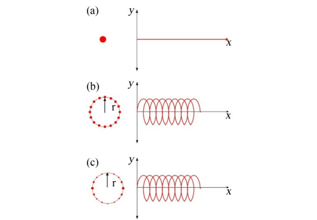
图3 不同激光加载模式扫描轨迹示意:(a)GHS-LW;(b)CPM-LW;(c)FDPM-LW
