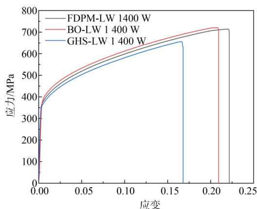
图 19 不同加载模式下 Inconel 625 焊接接头应力-应变曲线
