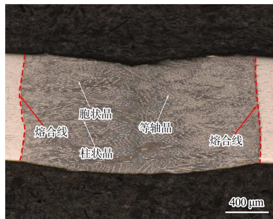
图 10 CPM-LW 焊缝截面金相组织
