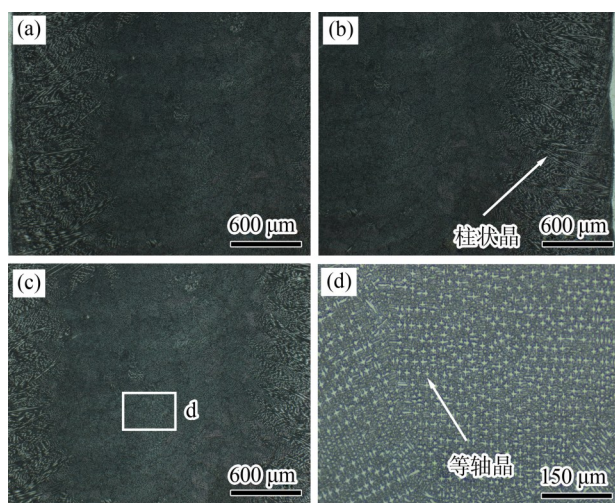
图 13 FDPM-LW 焊缝表面金相组织: (a) 焊缝左侧; (b) 焊缝右侧; (c) 焊缝中心; (d) 焊缝中心等轴晶
