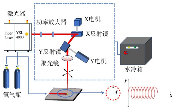
图1 激光焊设备示意
