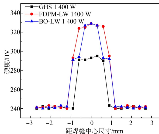
图 21 三种激光模式焊接接头硬度分布
