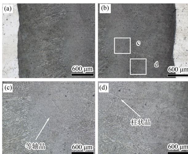
图 11 CPM-LW 焊缝表面金相组织: (a) 焊缝左侧; (b) 焊缝右侧; (c) 焊缝中心等轴晶; (d) 焊缝右侧柱状晶
