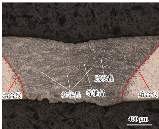
图 8 GHS-LW 焊缝截面金相组织
