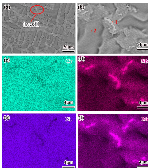
图 15 GHS-LW 焊缝区析出相 SEM 图像
