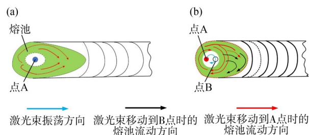
图 6 熔池和熔体流动示意:(a)无振荡;(b)圆周振荡
