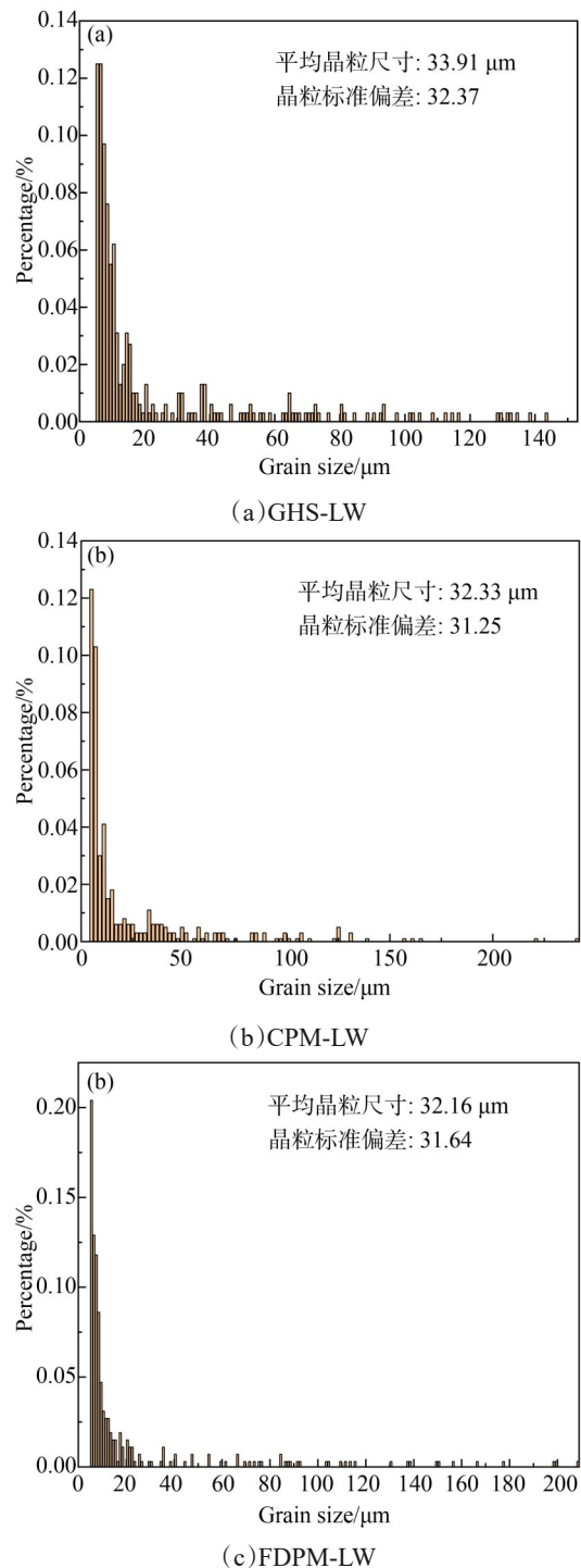
图18 不同加载模式的Inconel 625焊缝中心区域晶粒统计 Fig. 18 Grain statistics of Inconel 625 weld center region in different imposition modes
