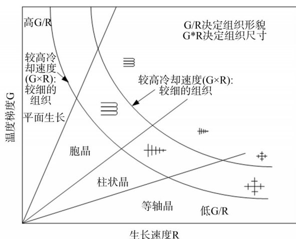
图 7 温度梯度 G 、生长速率 R 对凝固组织形态和速率的影响
