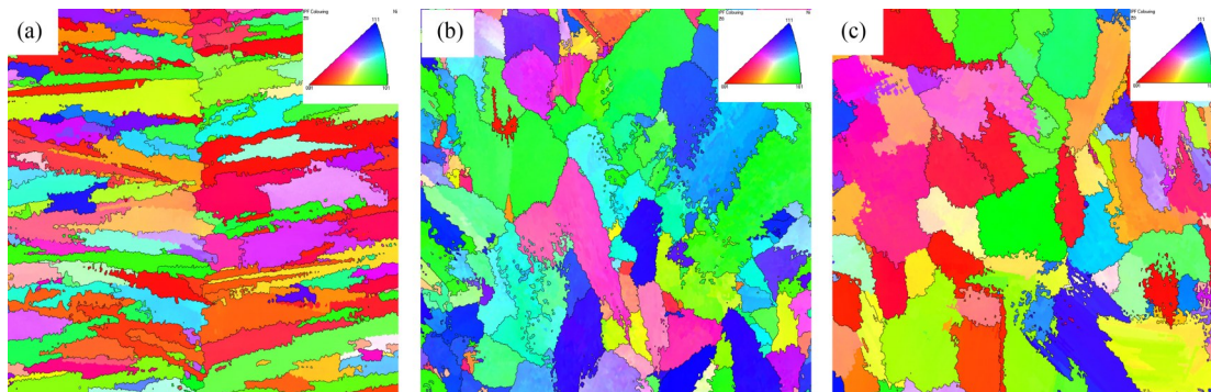
图 17 不同加载模式下的 Inconel 625 焊缝中心区域晶粒取向分布: (a)GHS-LW; (b)CPM-LW; (c)FDPM-LW
