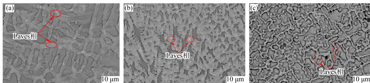
图 16 不同加载模式下 Laves 相的形态分布: (a)GHS-LW; (b)CPM-LW; (c)FDPM-LW
