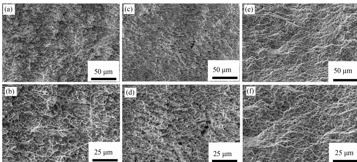
图 20 不同加载模式下 Inconel 625 拉伸试件断口 SEM: (a,b) GHS-LW; (c,d) CPM-LW; (e,f) FDPM-LW
