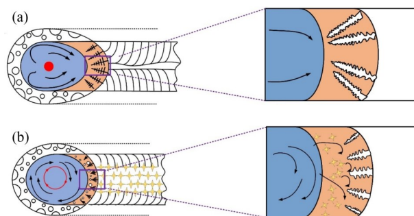
图 14 熔池流动对微观组织影响示意: (a) 无光束振荡; (b) 有光束振荡
