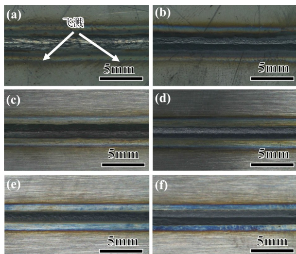
图 5 不同加载模式焊缝表面成形:(a)GHS-LW 正面;(b)GHS-LW 背面;(c)CPM-LW 正面;(d)CPM-LW 背面;(e)FDPM-LW 正面;(f)FDPM-LW 背面
